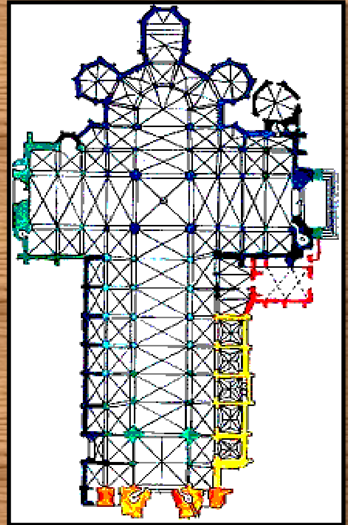
Plan de la cathédrale de Saint Omer
